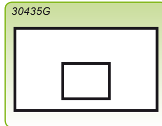
30435G Basketbord polyester Bord met een multiplex kern, afgewerkt met een met glasvezel versterkt polyesteren buitenlaag (dikte 22 mm). Voorzien van zwarte rand- en doelmarkering. Geschikt voor indoor- en outdoorbasket. 30435G Basketbord polyester 180 x 105 cm € 275,00
